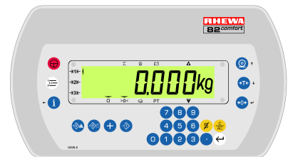
Rhewa 82 C1 mit Zehner-tastatur zur Eingabe von Soll- und Tarawerten
